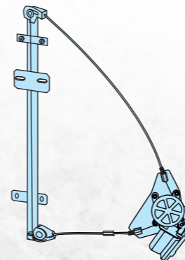
CF0/176 d-rh-rechts CF0/176 s-lh-links elettrico con motorino, 6 PIN electric with motor, 6 PIN elektrisch mit Motor, 6 PIN
