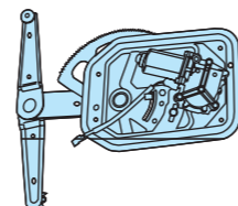
OFH/164 d-rh-rechts OFH/165 s-lh-links elettrico, con motorino electric, with motor elektrisch, mit Motor
