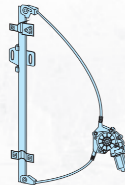
CF0/174 d-rh-rechts CF0/175 s-lh-links elettrico con motorino electric with motor elektrisch mit Motor
