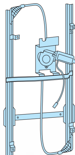
385/174 d-rh-rechts 385/175 s-lh-links elettrico con motorino electric with motor elektrisch mit Motor
