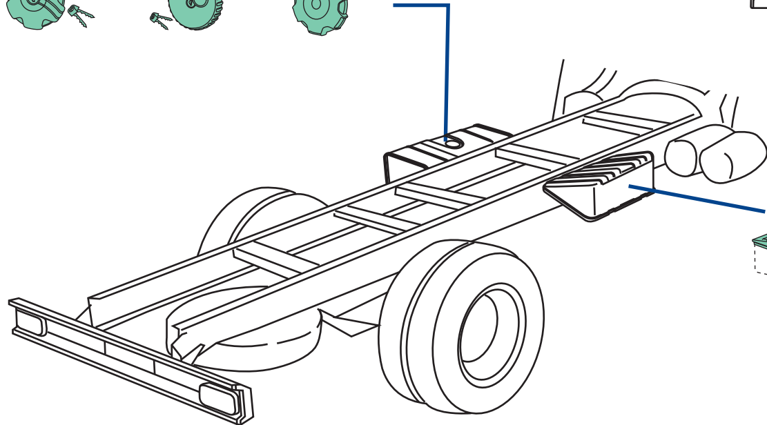
XF0/670
