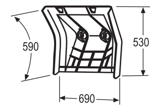
2FH/518
