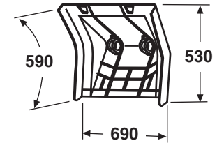
2FH/518
