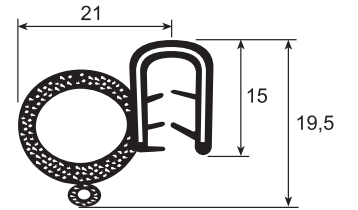
OFH/190
